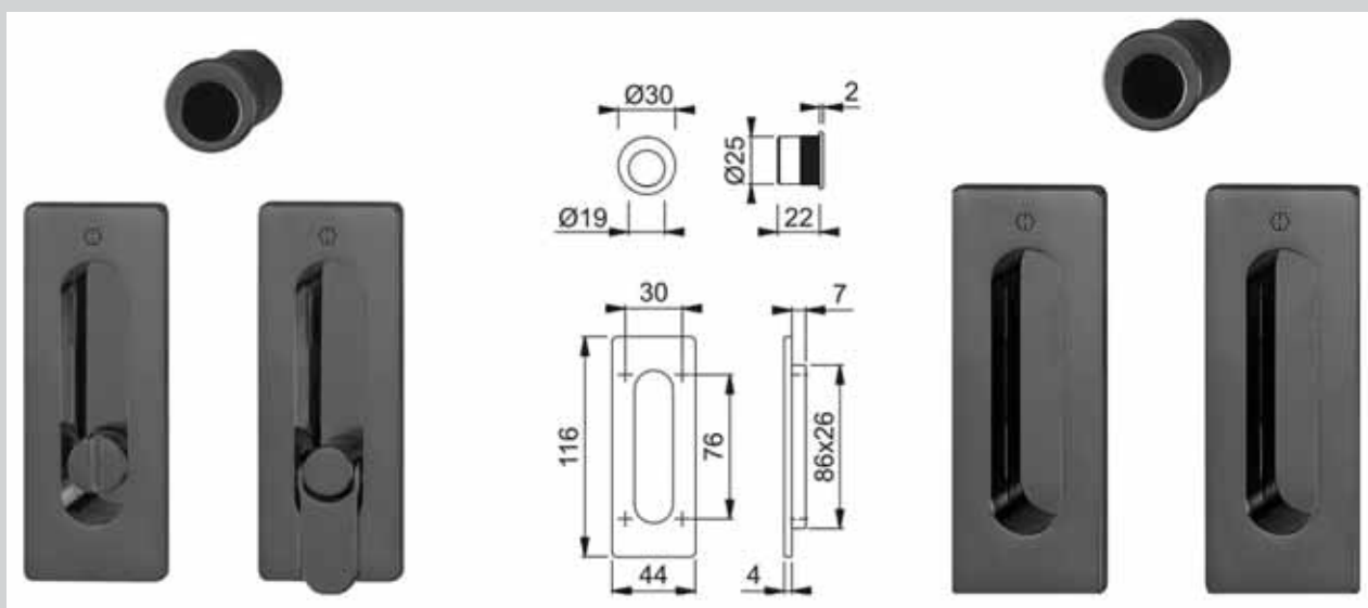
Set utopnih ročajev v paru, v obdelavi črna mat z naprstnikom za drsna lesena vrata
